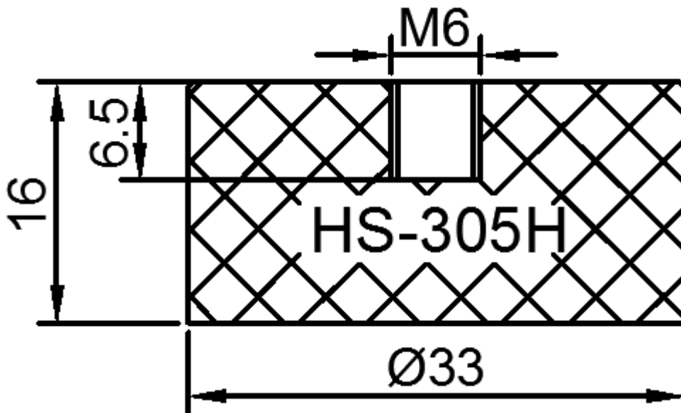
外形尺寸图
