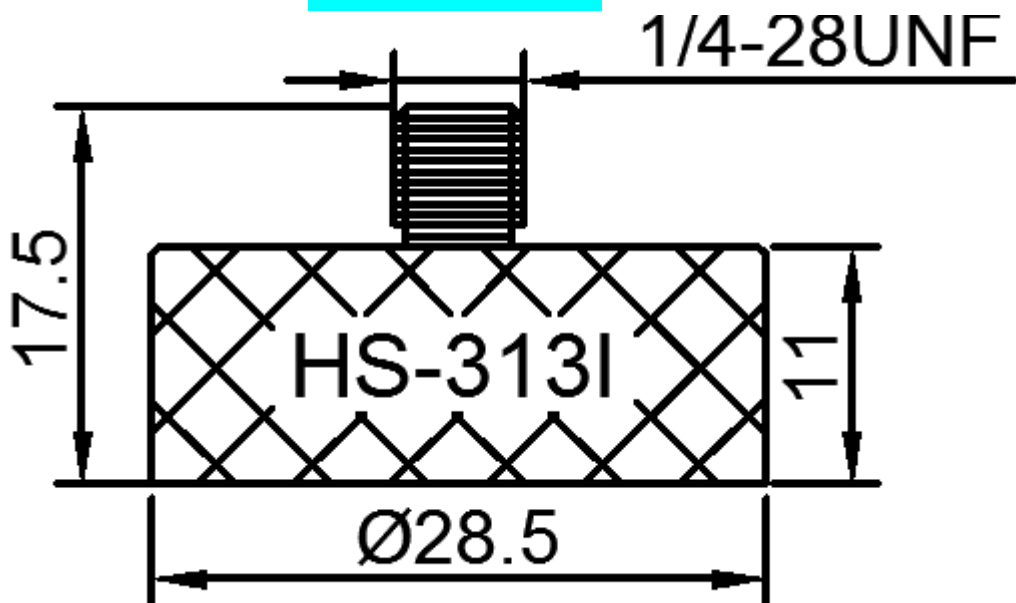
外形尺寸图
